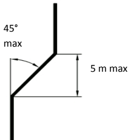
Dévoisement des conduits de fumée.
