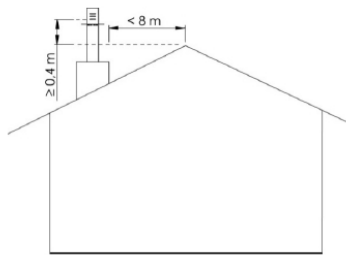
Sortie de fumée en Zone 1 dépassant de 40 cm au dessus du faîtage.
