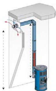
Evacuation des fumées en façade
